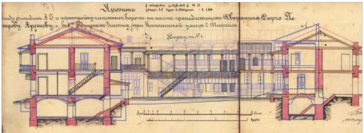
ნახ. 7. გ.აბესაძის ქ. №21 ნაგებობათა შეთავსებული გრძივი ჭრილები: 1881 წლის პროექტის და რეაბილიტაციამდე არსებული მდგომარეობის მიხედვით, 2024
