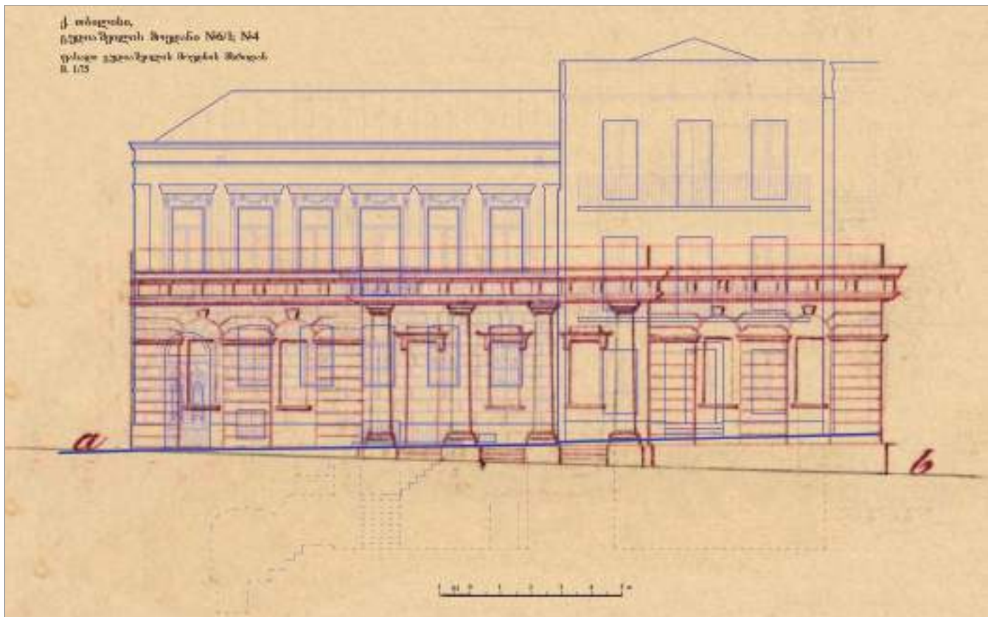
სურ.46. ლ. გუდიაშვილის მოედანი №6/1 და 4 საცხოვრებელი სახლების ფასადების არსებული მდგომარეობა და ამ ადგილზე XIX ს-ის დასაწყისში მდებარე ჰაუპტვახტის შენობის ფასადი საარქივო დოკუმენტის მიხედვით.
