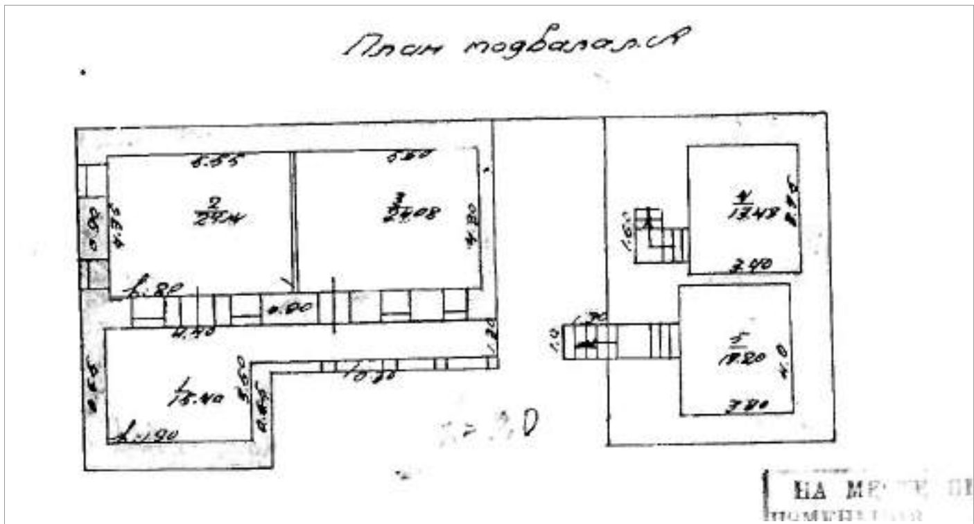
ნახ. 1. ბ. ახოსპირელის III ჩიხი №1/17, ტექ.ბიუროს ნახაზი, სარდაფის სართული, 1960-იანი წლები
