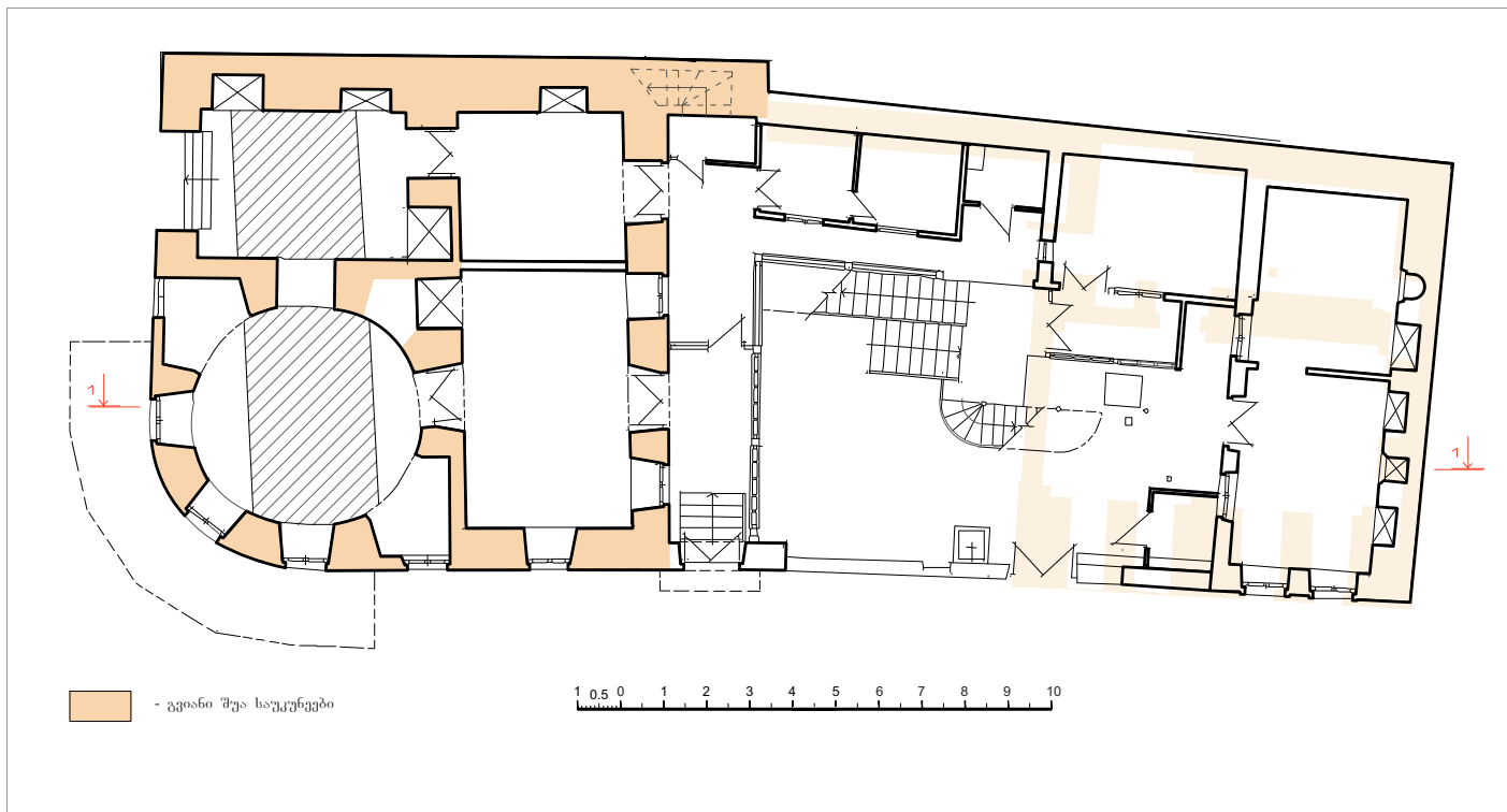
ნახ. 2. №34/17 სახლის I სართულის გეგმა
