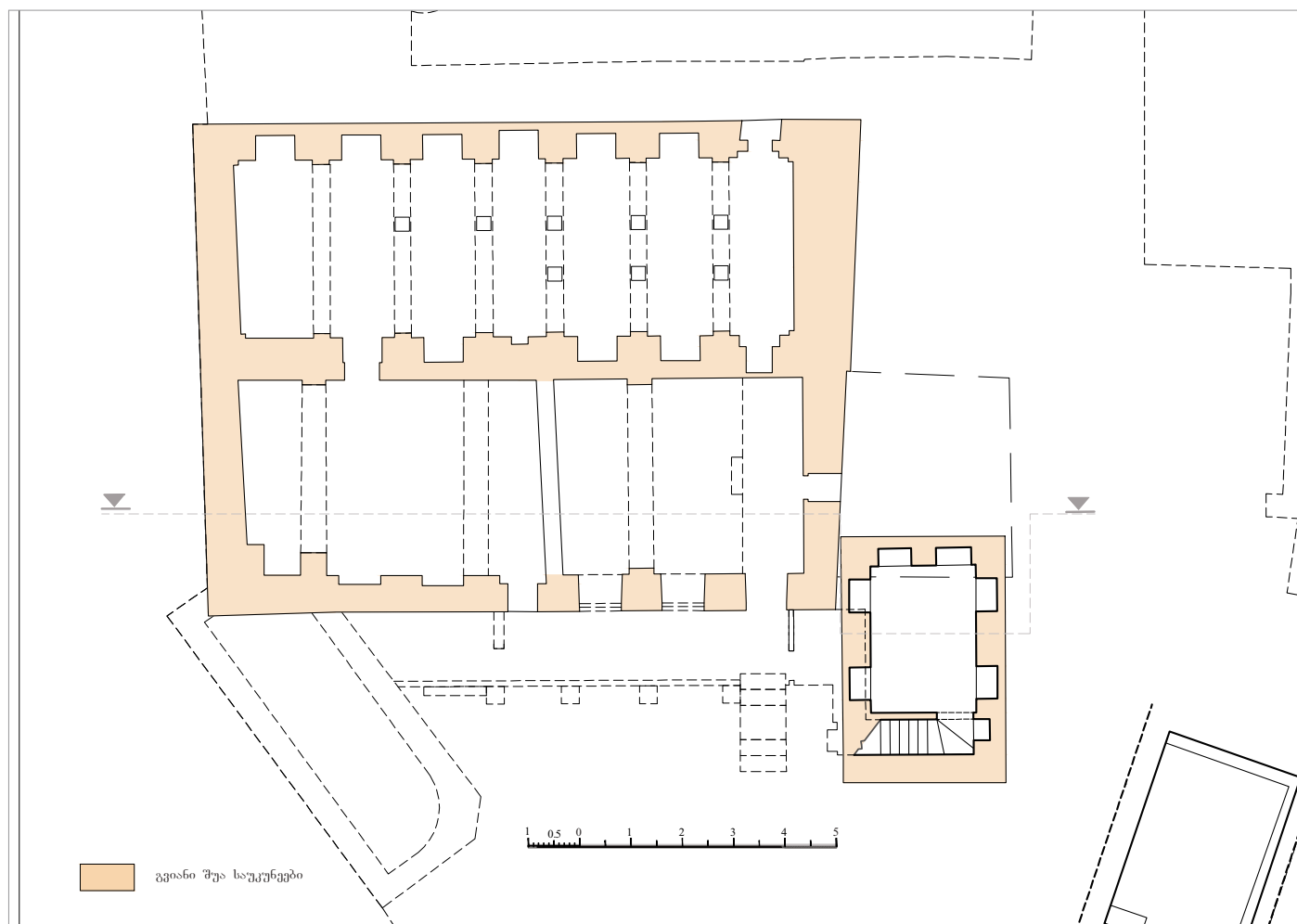
ნახ. 1. აბო თბილელის ქ. №6, სარდაფის გეგმა
