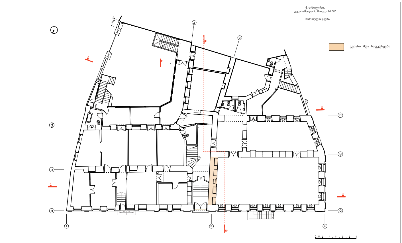
ნახ. 1. ლ. გუდიაშვილის მოედანი №7/3 და №2/7 შენობების I სართ. გეგმა
