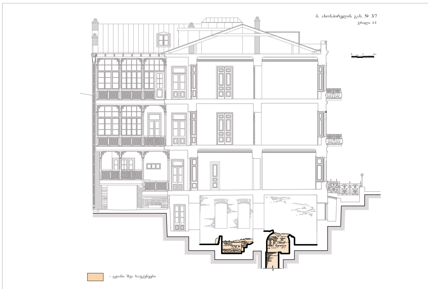
ნახ. 2. ბ. ახოსპირელის გასასვლ. №3/7, შენობის ჭრილი ძველ ნაგებობათა ნანგრევების ჩვენებით
