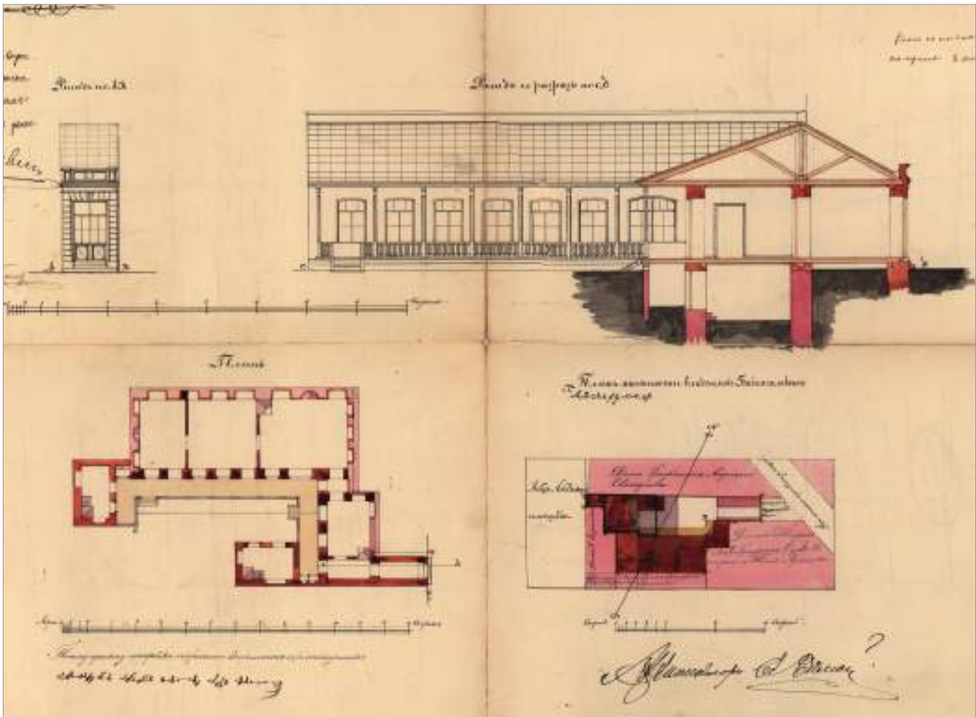
სურ. 1. საისტორიო ცენტრალური არქივი, ფონდი №201, ანაწერი №1, დოკუმენტი №2744, საცხოვრებელი სახლის პროექტი
