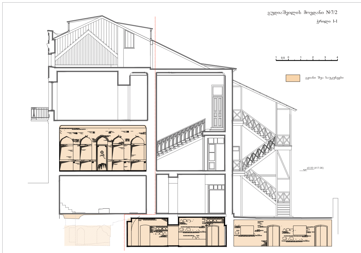
ნახ. 3. ლ. გუდიაშვილის მოედანი №7/2, განივი ჭრილი ძველი ფენების ჩვენებით
