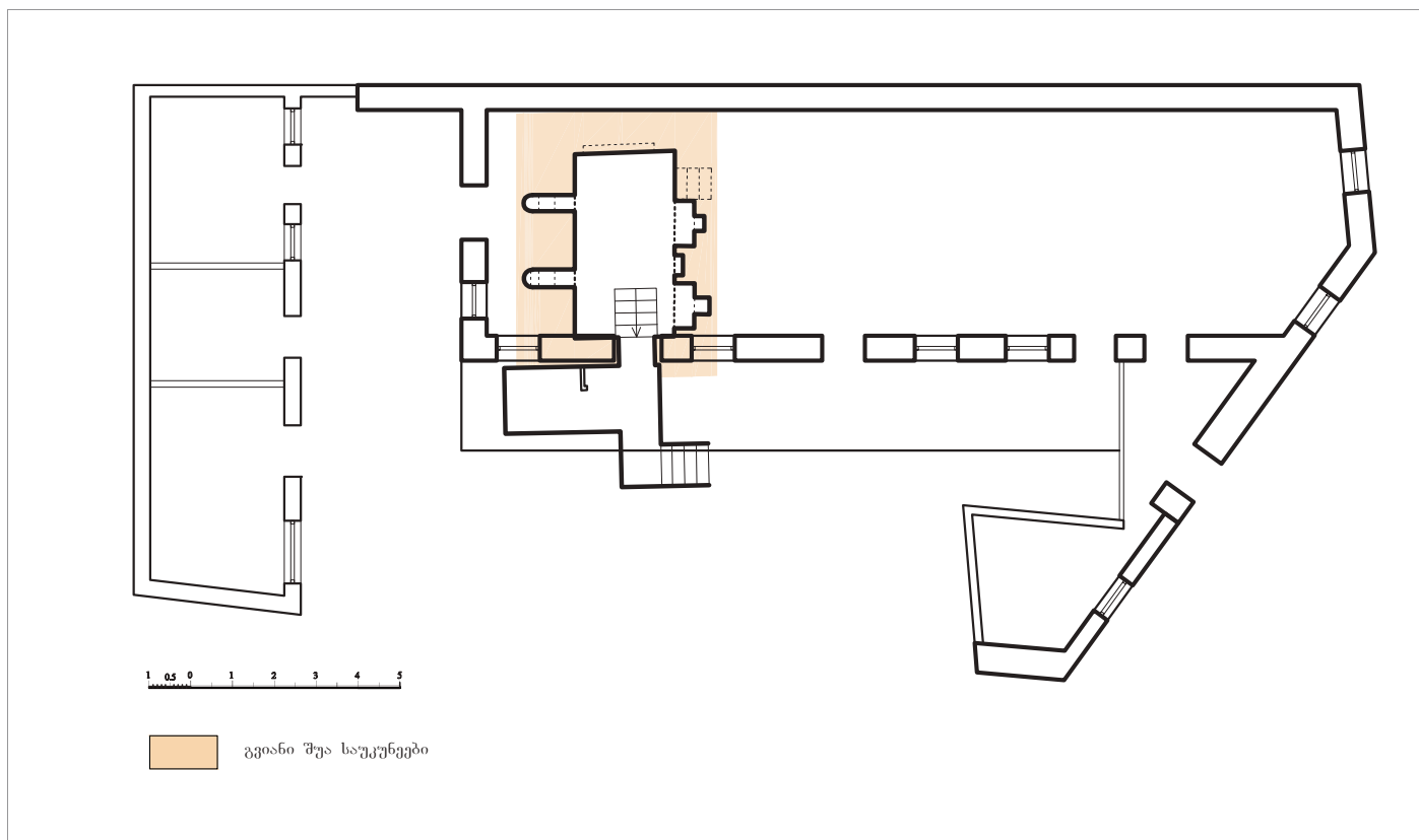
ნახ. 1. ბ. ახოსპირელის III ჩიხი №9, სახლის გეგმა ძველი სარდაფის ჩვენებით.
