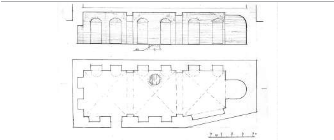
ნახ.2. სიღნაღი, ც.დადიანის და ვ. სარაჯიშვილი ქუჩების შესაყარი, ღვინის სარდაფი, გვგმა, ტბილი.
