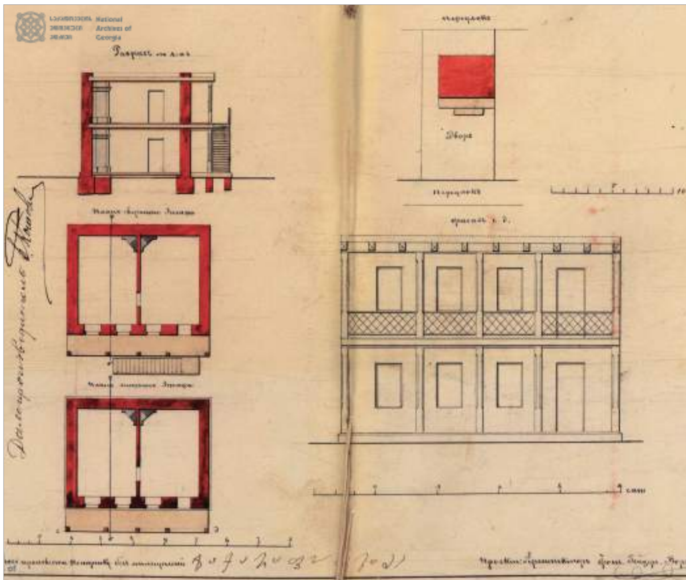
ნახ. 1. გორის მცხოვრებ ზაქარია ფოფხაძის ორსართულიანი სახლის პროექტი მიწის სახურავით. 1881. არქიტექტორი ფონ ჰეიდერ ბოროვსკი
