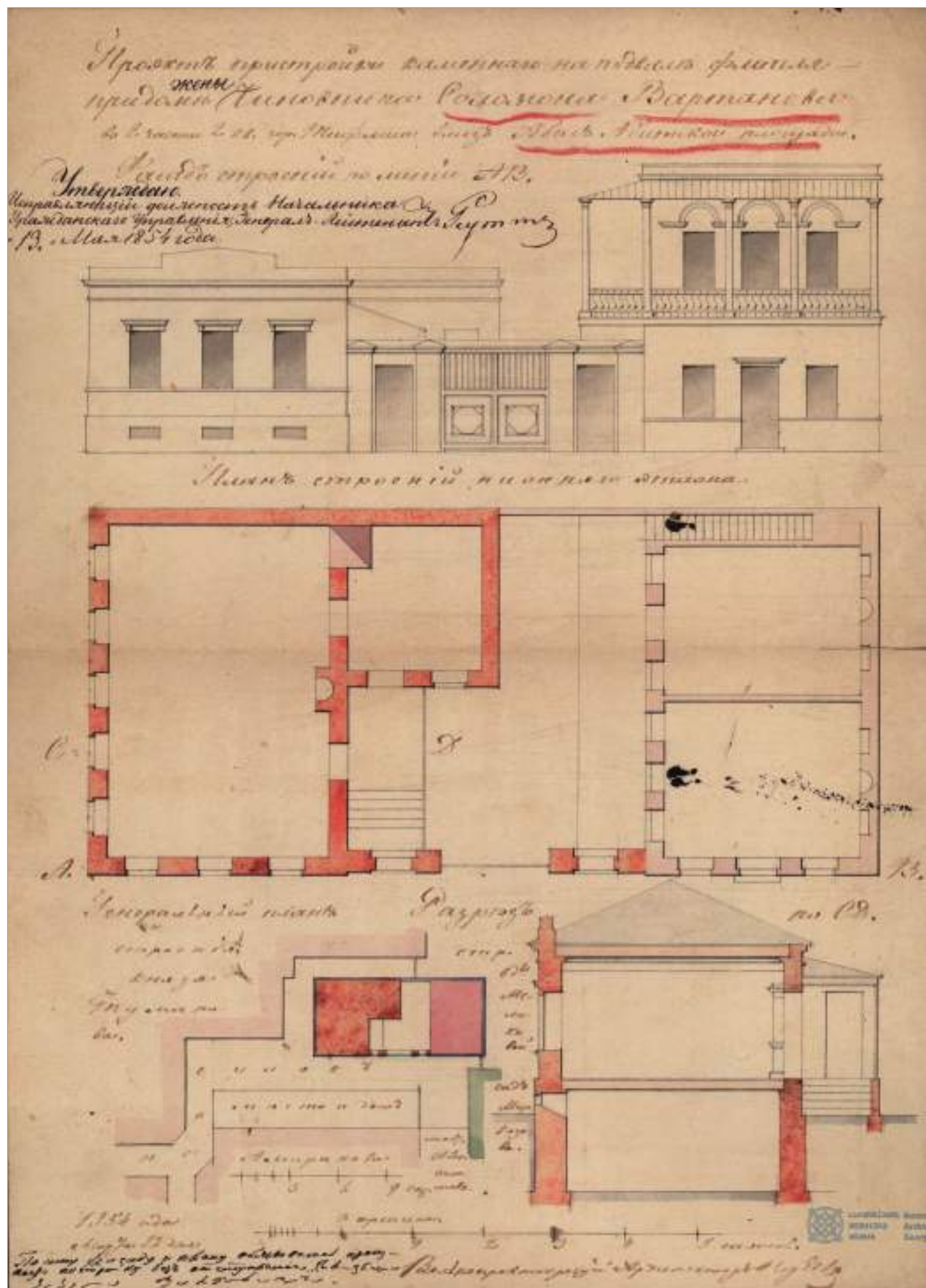
ნახ. 2. კეკელა ვართანოვას სახლის მიწეუბნის პროექტი, 1854
