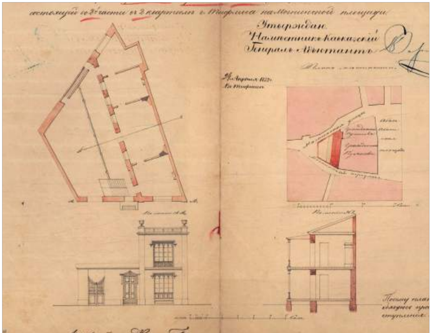
ნახ. 2. კნიაგინია ბეგთაბეგოვას ორსართულიანი სახლის პროექტი, 1859
