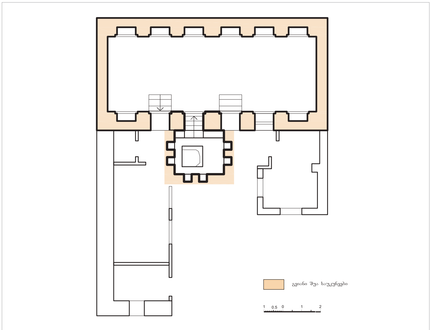
ნახ.1. გ.ჭიბლაძის ქ.№3, ორსადგომიანი სარდაფის გეგმა
