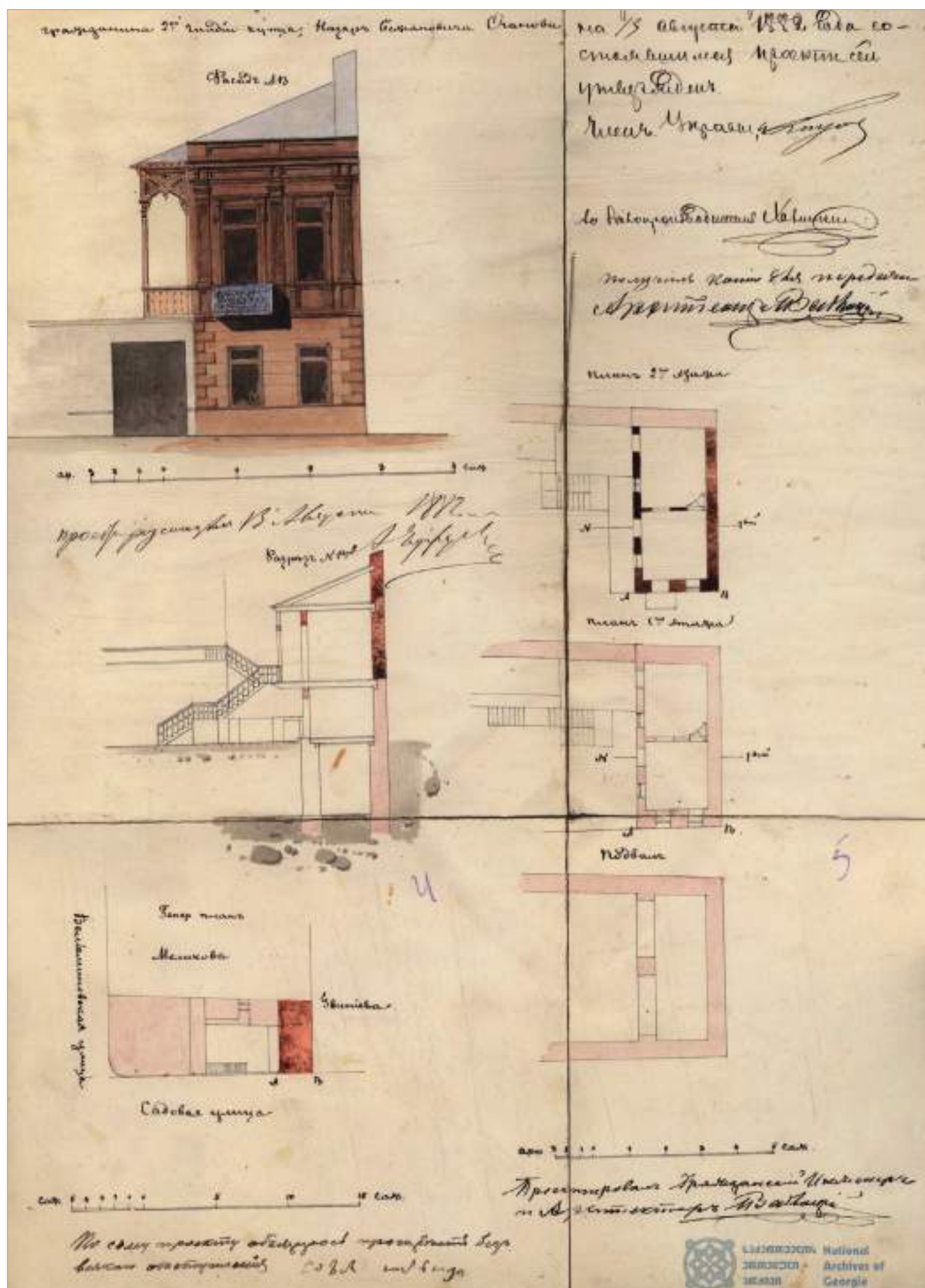
ნახ. 4. ნაზარ ოგანოვის სახლის საარქიტექტო პროექტი, 1882
