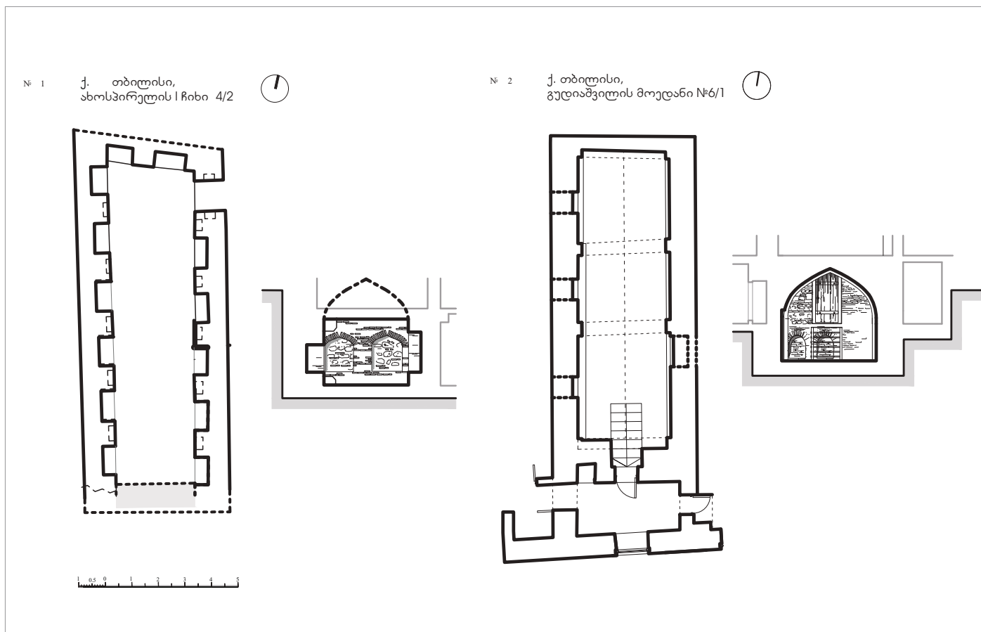
ნახ. 5. ბ. ახოსპირელის I ჩიხი, საცხოვრებელი სახლი №4/3, ახლად გამოვლენილი სადგომის გეგმის რეკონსტრუქცია და ლ.გუდიაშვილის მოედანი №6/1 საცხოვრებელ სახლში შემონახული ძველი სათავსის გეგმის არსებული მდგომარეობა.
