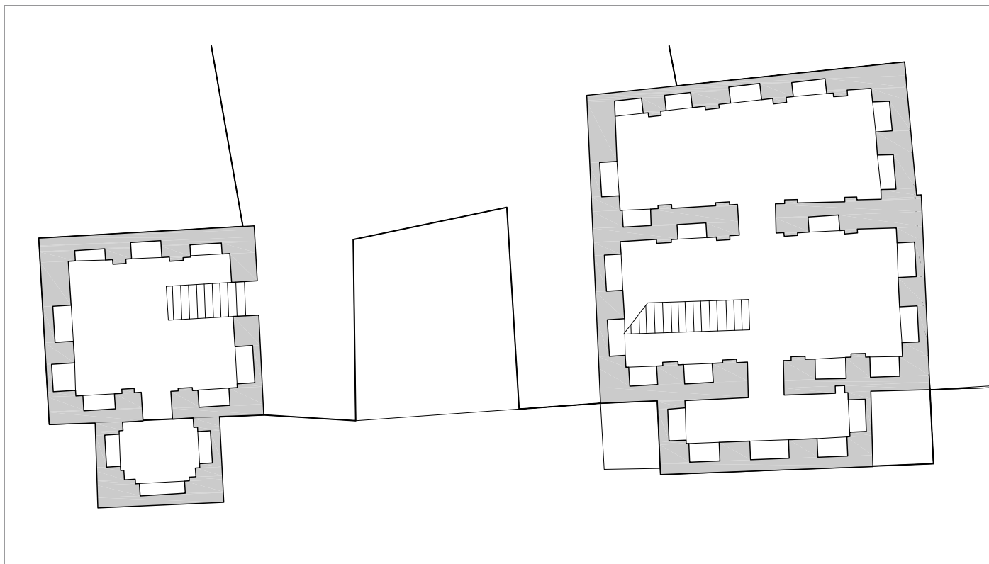
ნახ.1. ლ. გუდიაშვილის მოედანი, საცხოვრებელი სახლი №2, სარდაფის სართული, გეგმა.
