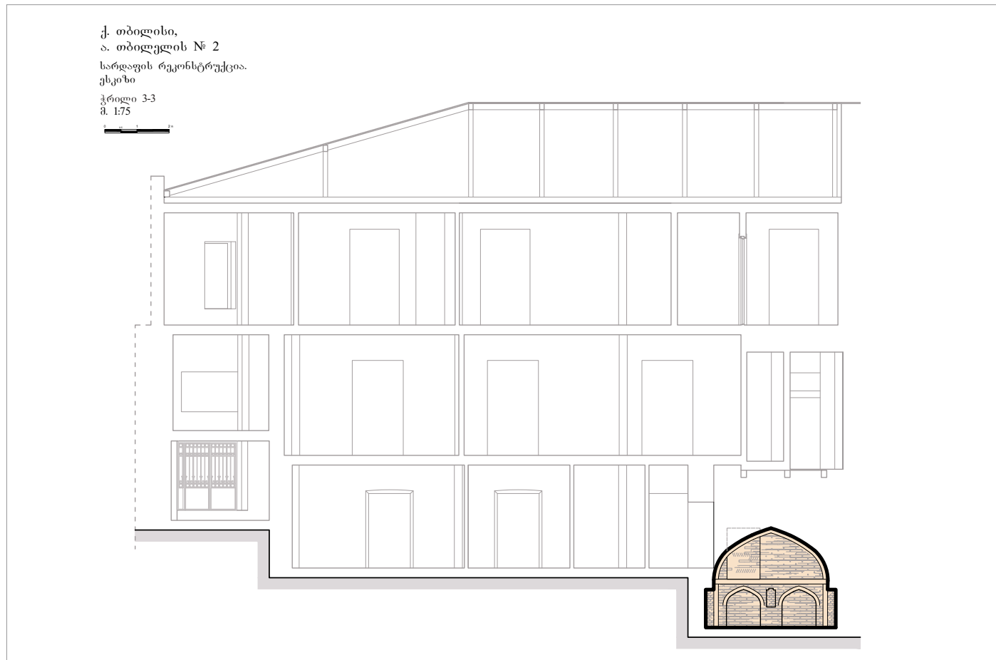
ნახ. 2. აბო თბილელის ქ. №2, საცხოვრებელი სახლის ჭრილი სარდაფის სადგომის ჩვენებით
