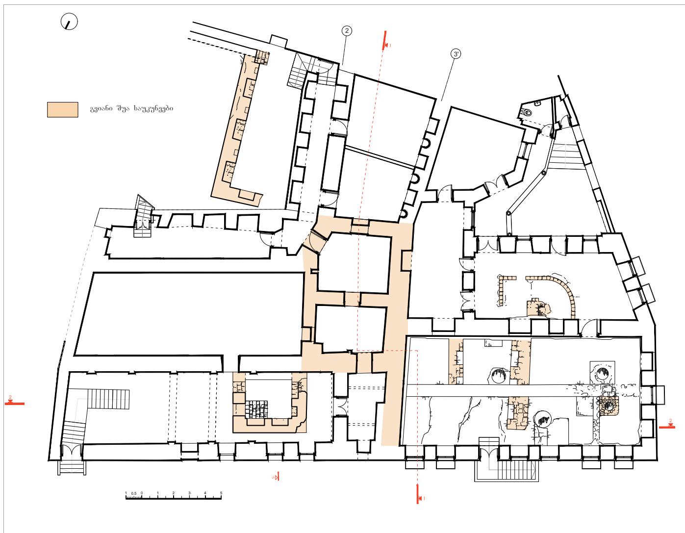
ნახ. 4. ლ. გუდიაშვილის მოედანი №7/2 და №7/3, სარდაფის სართული, არქეოლოგიური ფენები
