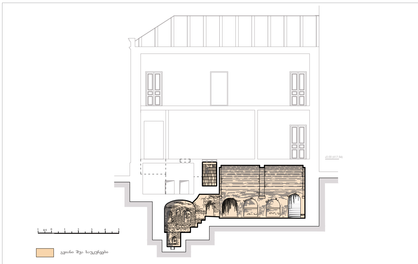
ნახ. 6. ლ. გუდიაშვილის მოედანი, საცხოვრებელი სახლი №6/1, ქვედა დონის სადგომის გრძივი ტრილი, ხედი დასავლეთით.
