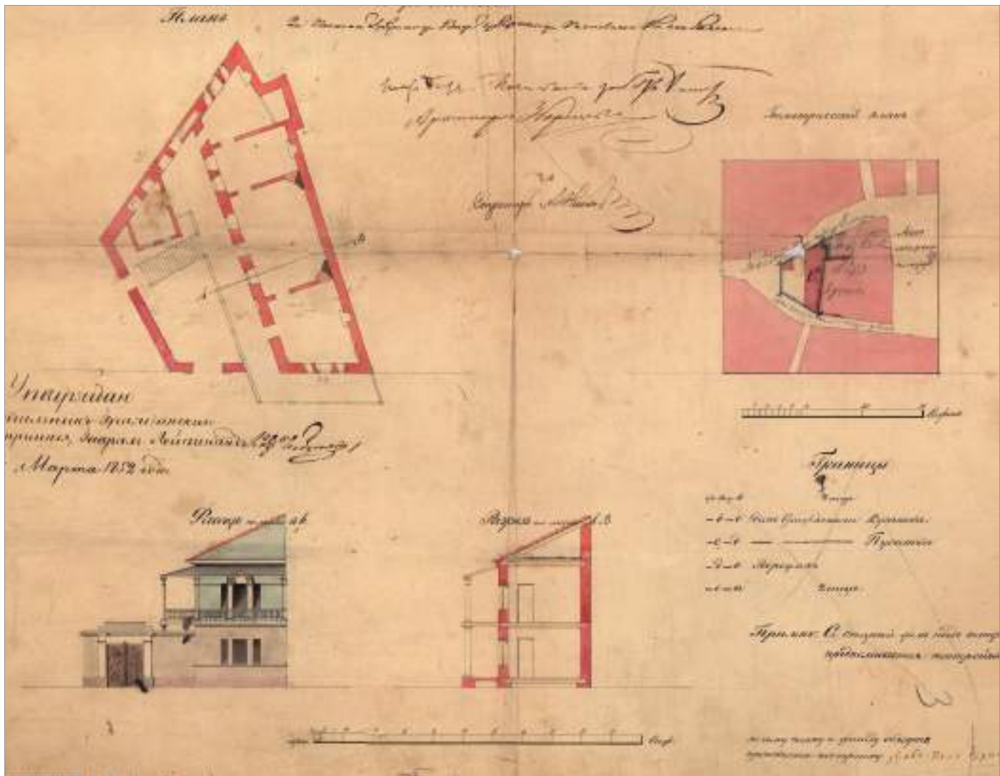
ნახ. 1. მარია ბეგთაბეგოვას სახლზე მეორე სართულის დაშენების პროექტი, 1852
