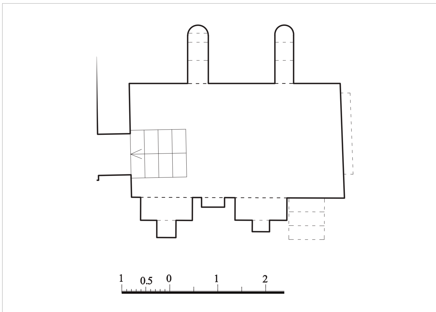
ნახ. 1. ბ. ახოსპირელის III ჩიხი №9, ძველი სარდაფის გეგმა
