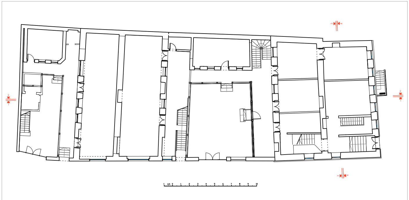
ნახ.1. ლ. გუდიაშვილის მოედანი, საცხოვრებელი სახლი №6/1, პირველი სართულის გეგმა.
