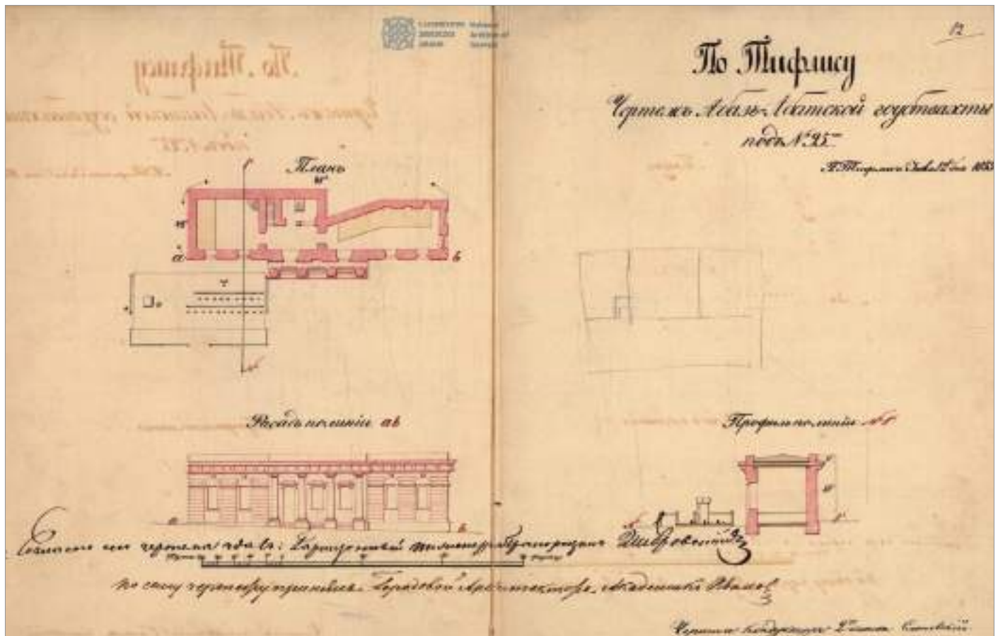
სურ.43. აბას-აბადის ჰაუპტვახტის შენობის გეგმა, ფასადი და ჭრილი, 1855-1856 წწ-ის საარქივო დოკუმენტი.
