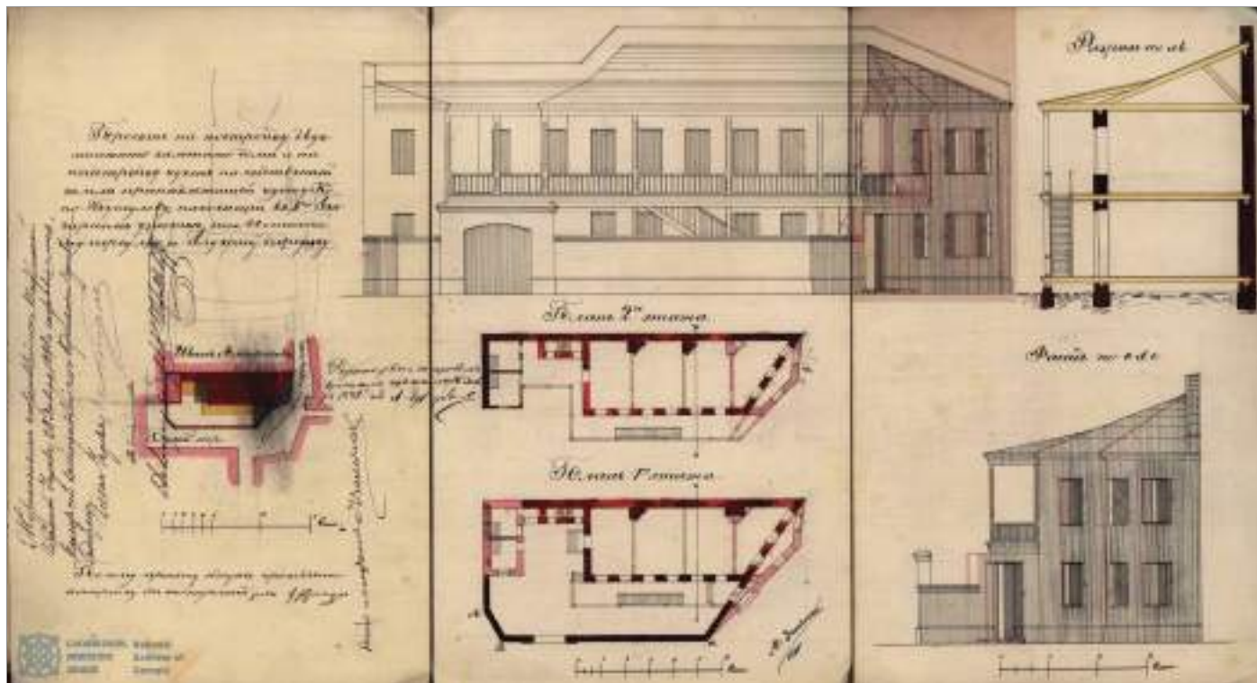
ნახ. 1. კონო ბუტულოვის სახლის პროექტი, 1881
