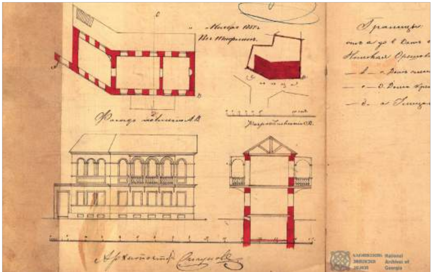
ნახ. 5. დავით არეშოვის სახლის პროექტი, 1857
