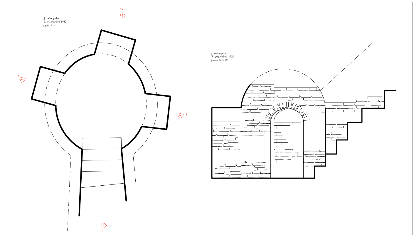
ნახ. 10. შ. დადიანის ქ. №32 სახლის ფუნდამენტის სივრცეში დაცული ძველი სათავსის გეგმა და ტრილი
