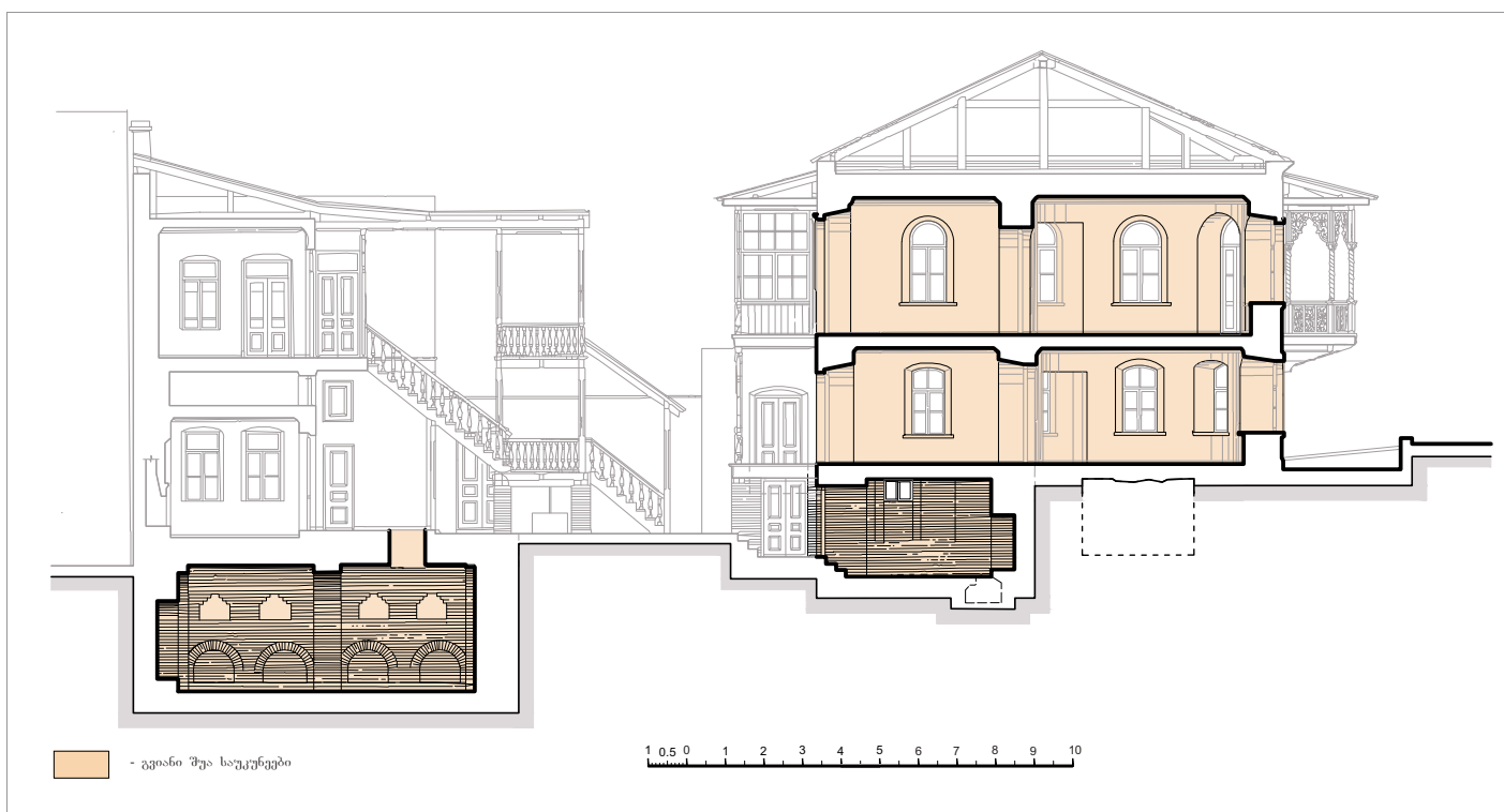
ნახ. 3. №34/17 სახლის ჭრილი.
