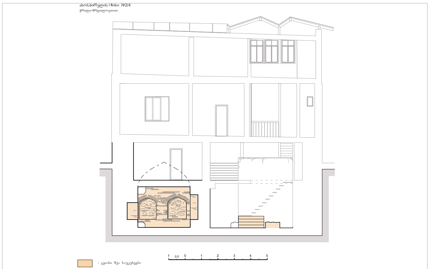
ნახ. 4. ბ. ახოსპირელის I ჩიხი, საცხოვრებელი სახლი №4/3, ახლად გამოვლენილი სადგომი, ტრილი, ხედი ჩრდილოეთით.
