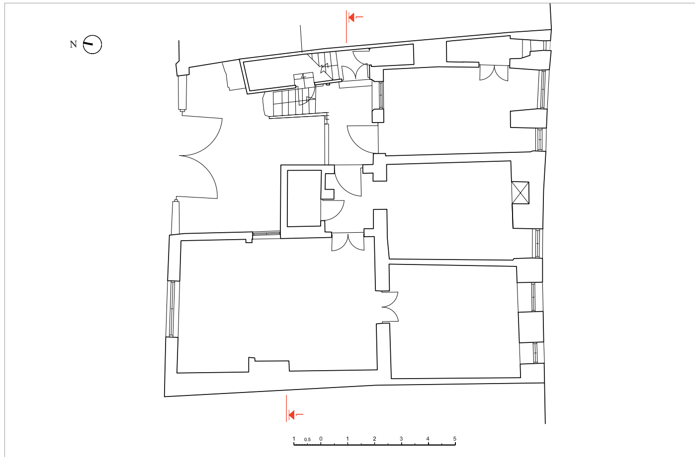
ნახ.2. ბ. ახოსპირელის I ჩიხი, საცხოვრებელი სახლი №4/3, პირველი სართული, გეგმა.
