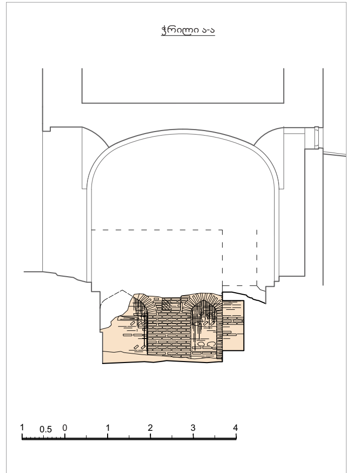
ნახ. 6. ლ. გუდიაშვილის მოედანი №7/3, სარდაფის ჭრილი XVII ს-ის ნაგებობის ნანგრევით
