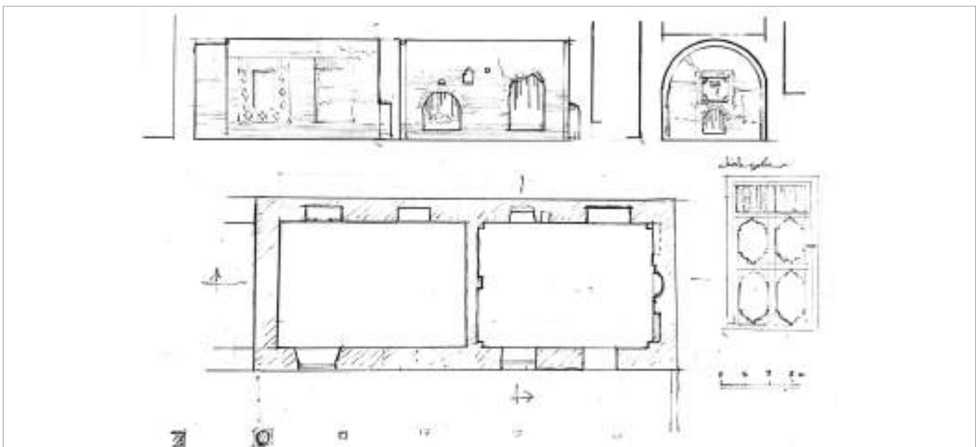
ნახ.3. სიღნაღი, თ. ჭილაძის ქ. №3, ღვინის სარდაფი, გვგმა, ტბილი, დეტალები.
