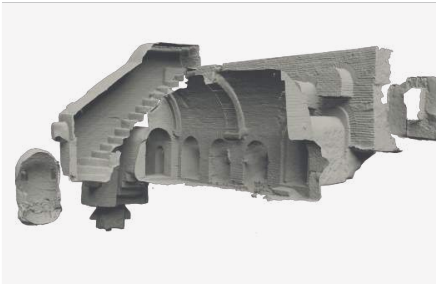
1. ფოტოგრამეტრიული 3D მოდელი, ლ.გუდიაშვილის მოედანი, საცხოვრებელი სახლი №6/1, ძველი შენობის ქვედა დონის სადგომის ინტერიერი, კიბე, და მიმდებარე სივრცე.
