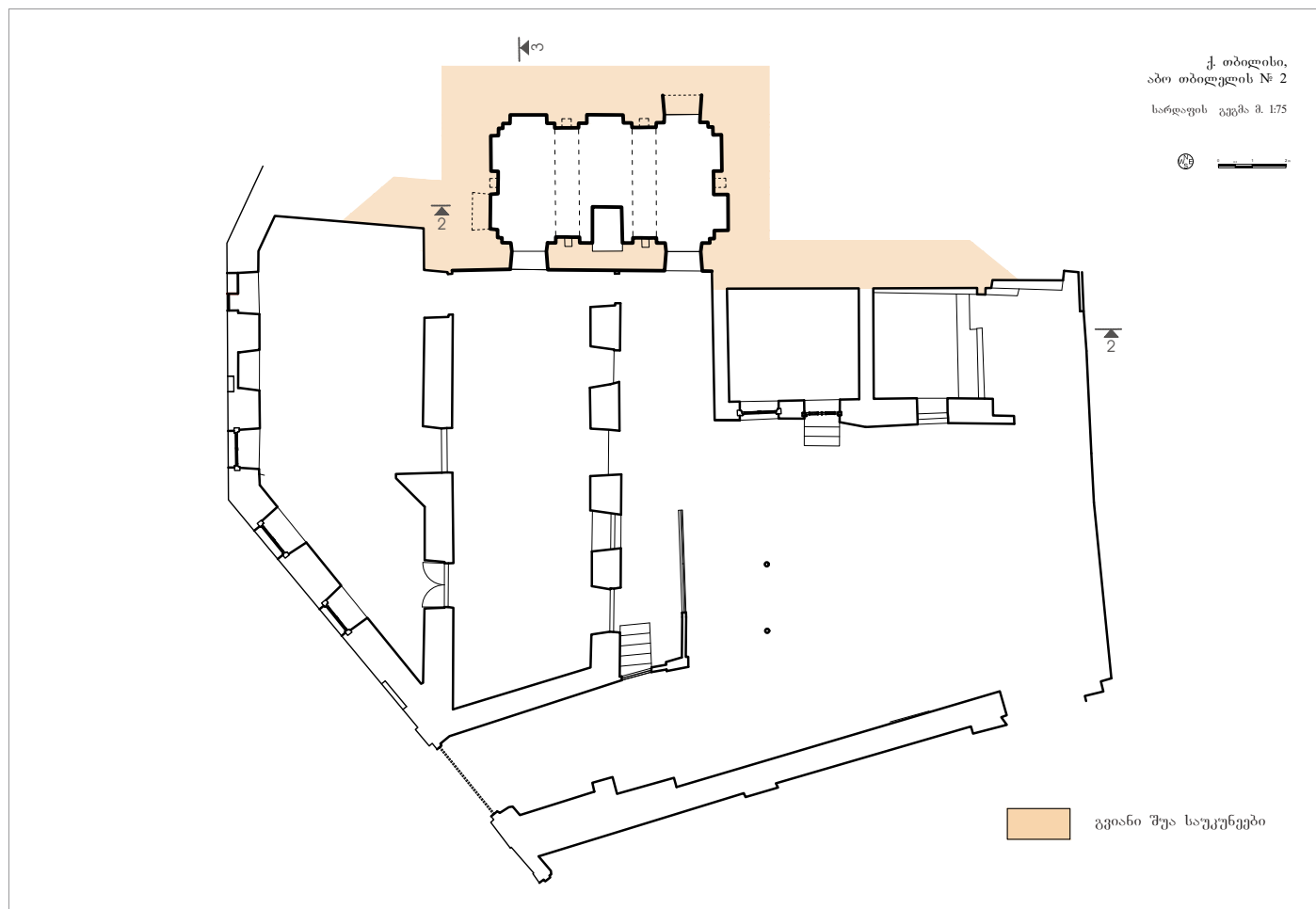
ნახ. 1. აბო თბილელის ქ. №2, საცხოვრებელი სახლის გეგმა სარდაფის სადგომის ჩვენებით
