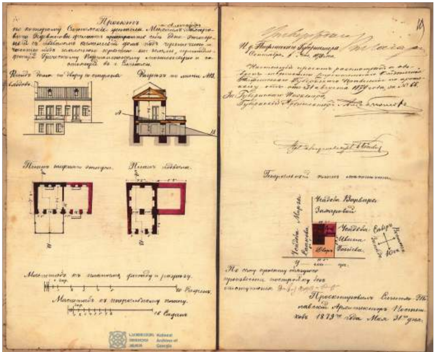
სურ.18. 1879 წლის პროექტი, ავტორი თელავისა და სიღნაღის არქიტექტორი პოსტნიკოვი, დოკუმენტი ინახება საქართველოს ეროვნული არქივის ცენტრალურ საისტორიო არქივში.
