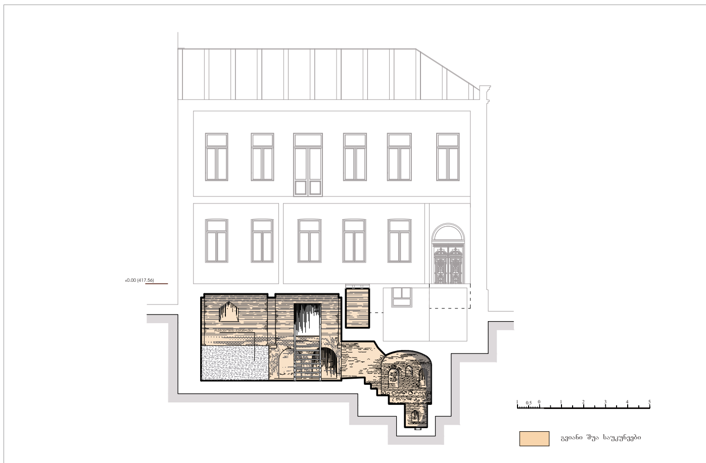
ნახ. 5. ლ. გუდიაშვილის მოედანი, საცხოვრებელი სახლი №6/1, ქვედა დონის სადგომის გრძივი ტრილი, ხედი აღმოსავლეთით.
