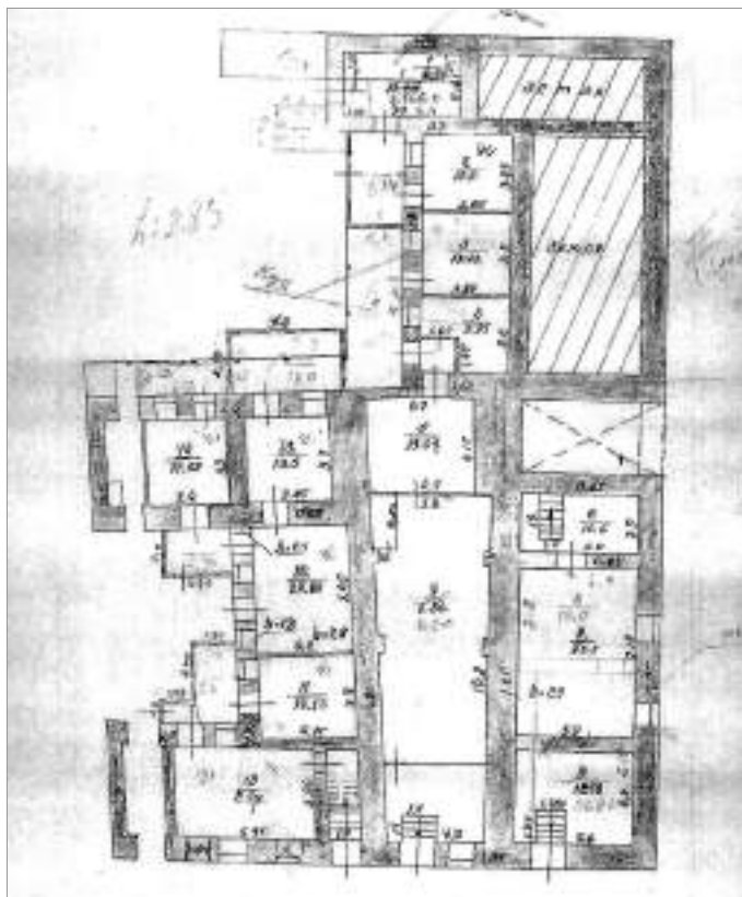
ნახ. 2. №20/6 სახლის ტექ.ბიუროს ანაზომი, სარდაფის სართულის გეგმა, 1957
