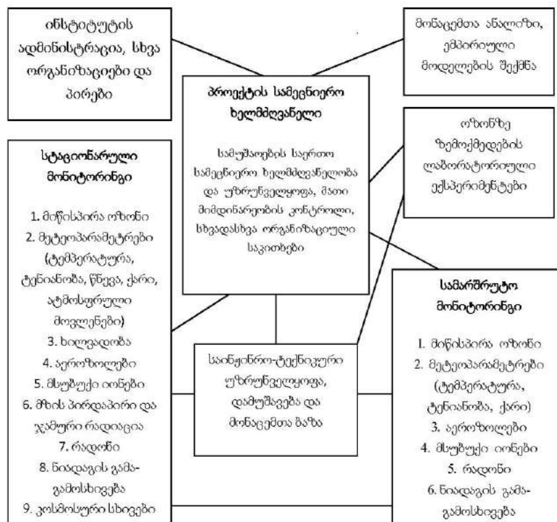
ნახ. 2.1 საველე და ლაბორატორიული ექსპერიმენტების ზოგადი სტრუქტურა
