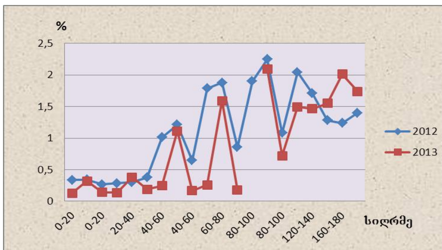
ნახაზი 4.1.5 მშრალი ნაშთის შემცველობა, % (წნორი, უდრენაჟო), 2012, 2013 წწ.
